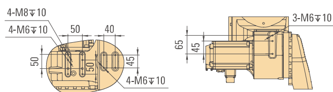
肘部孔位图 Elbow arm
