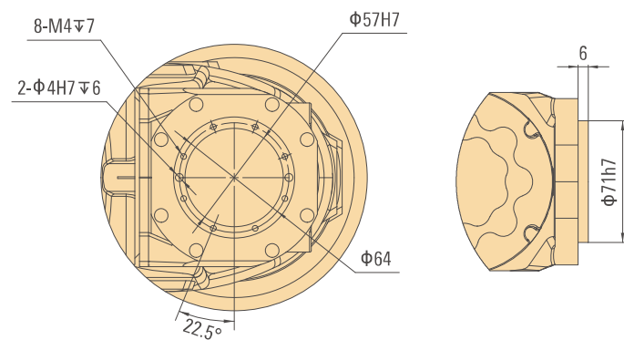
法兰图 Flange drawing
