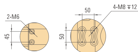
肘部孔位图 Elbow arm
