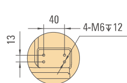
肘部孔位图 Elbow arm
