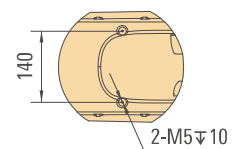
小臂孔位图 Upper arm
